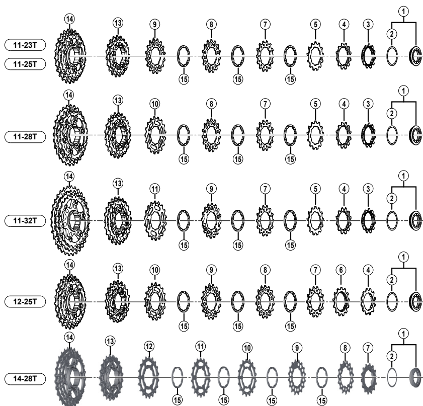
CS-6800 sprocket teeth combinations
