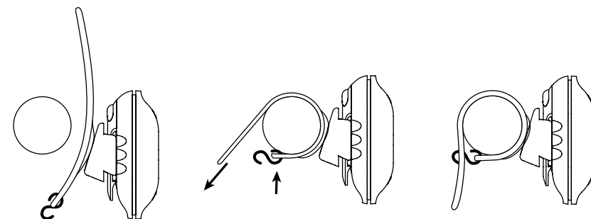
BLS-77 FRONTLASER
